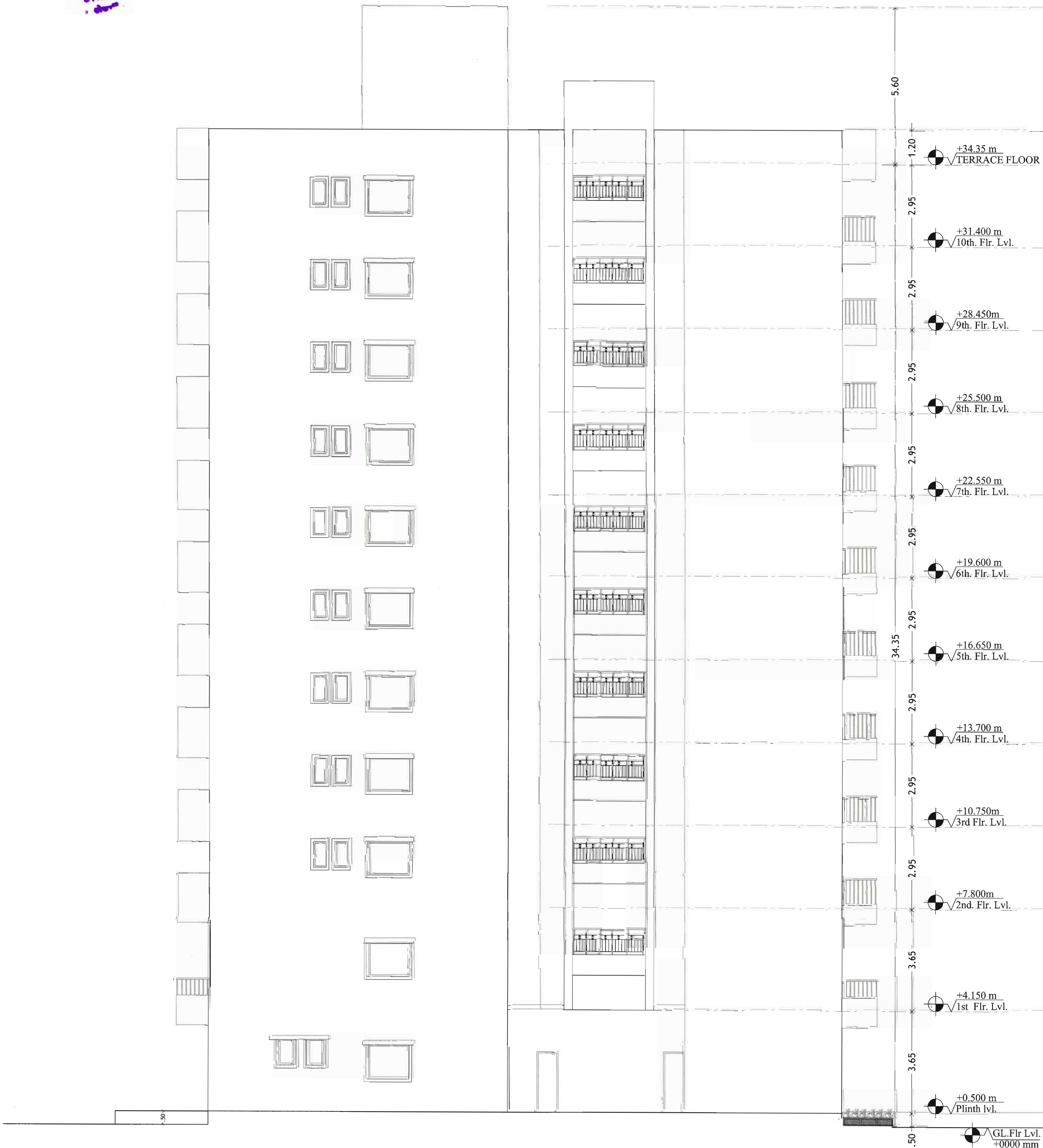
ELEVATION -A
